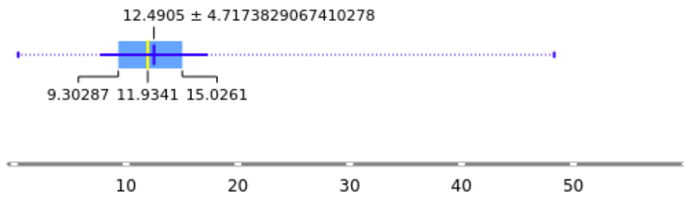
Figure 18: Distribution de la distance tumulus-alignement
