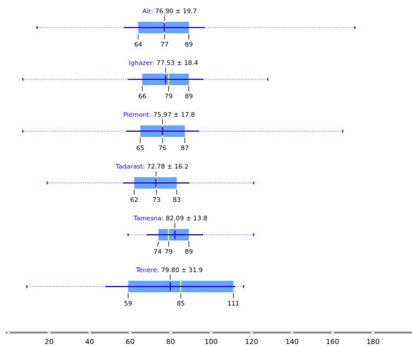
Figure 5: Moyenne et médiane de l'orientation par zone
