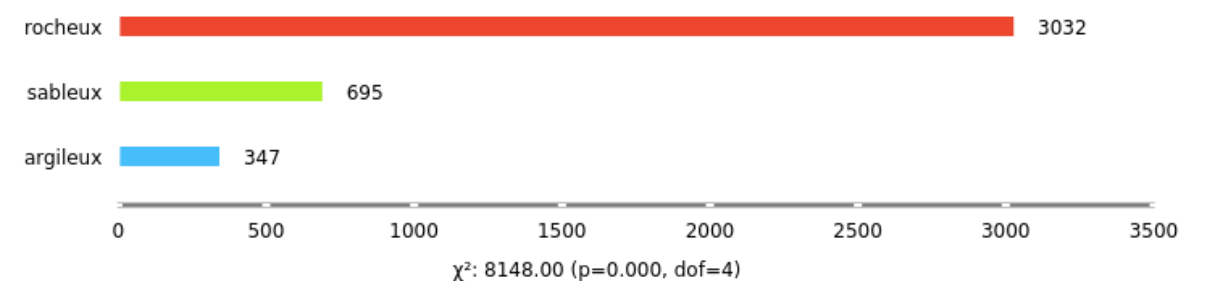
Figure 2: Nombre de monuments par types de support
