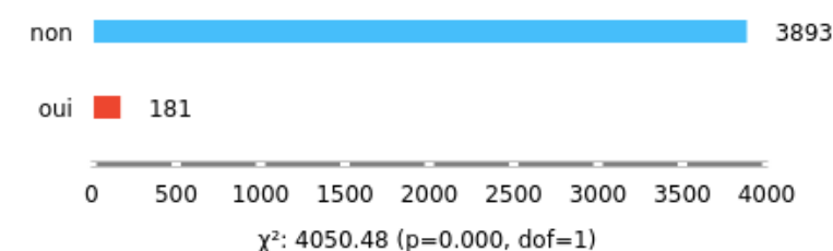
Figure 14: Nombre d'alignements avec un tumulus à l'extrémité
