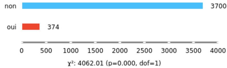
Figure 15: Nombre d'alignements dont la grosseur des tourettes augmente vers le sud
