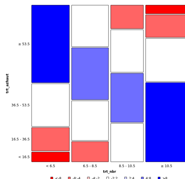
Figure 11: Mosaïque du nombre de tourette par rapport à l'Azimut haut
