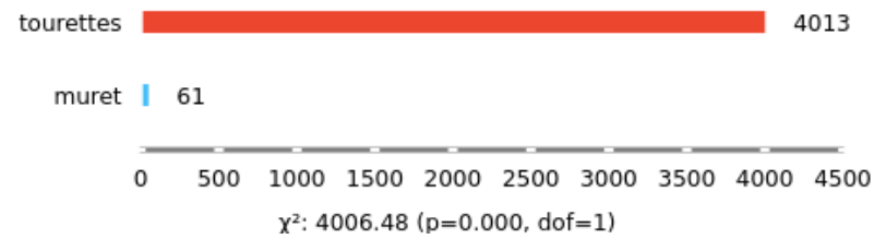
Figure 17: Nombre de monuments selon la composition de l'alignement
