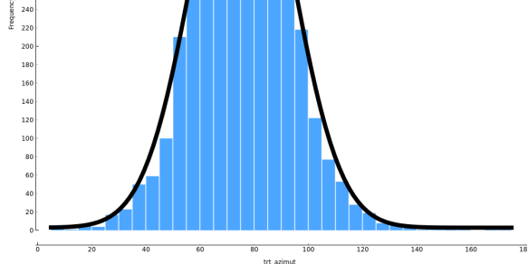
Figure 4: Distribution de l'orientation des monuments à alignement
