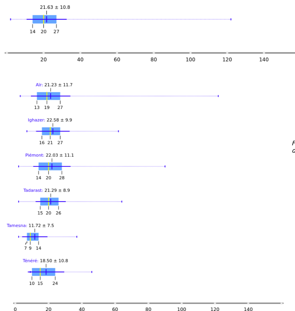
Figure 12: Moyenne et médiane de la longueur des alignements
