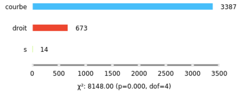
Figure 16: Nombre de monument selon la forme de l'alignement
