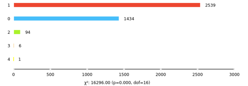
Figure 7: Nombre de monuments possédant un anneau de pierre
