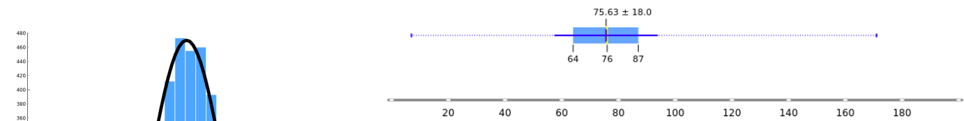
Figure 3: Moyenne et médiane de l'orientation
