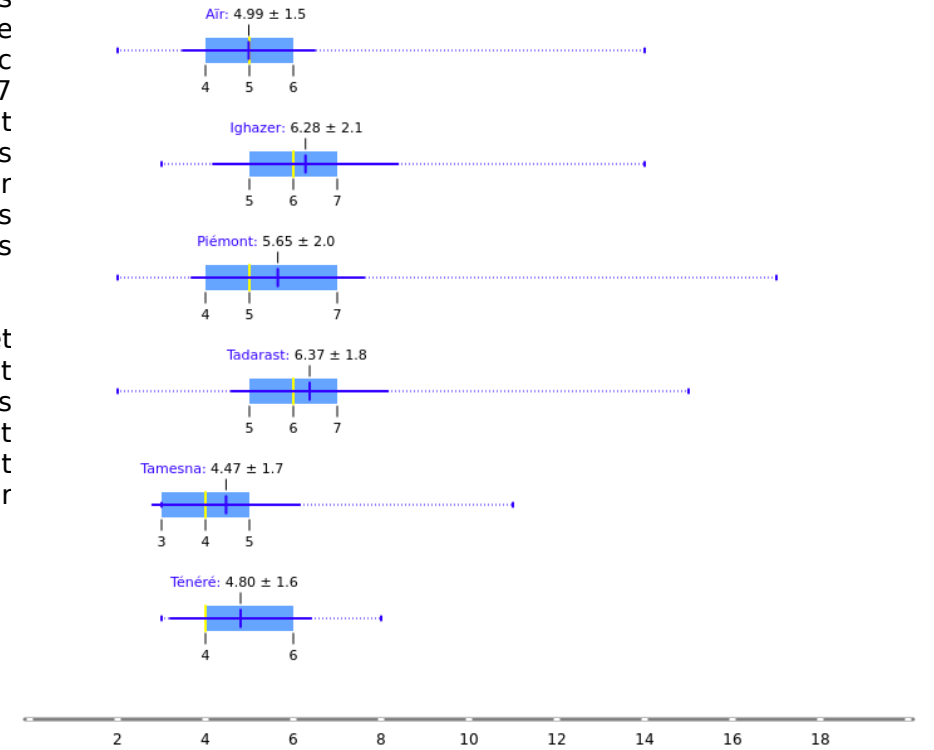
Figure 6: Distribution de la taille des monuments par zone géomorphologique
