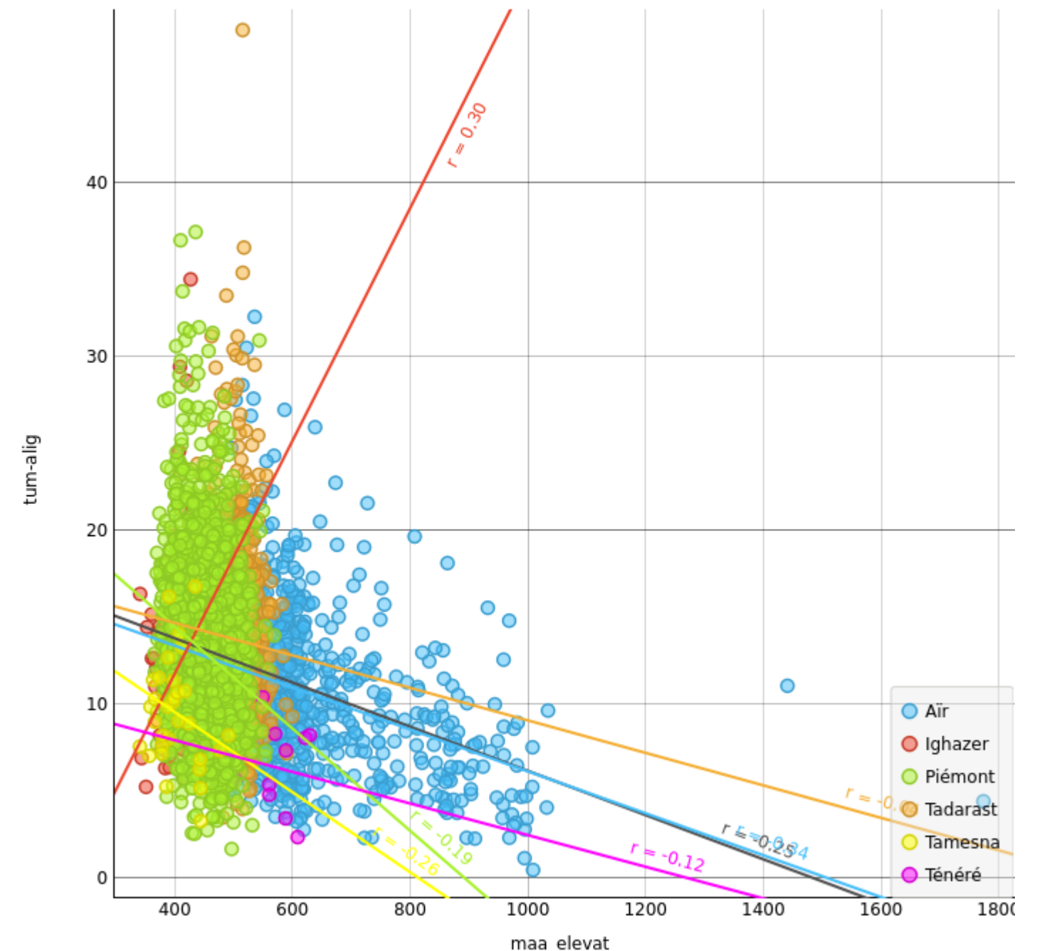
Figure 20: Distance tumulus-alignement en fonction de l'altitude
