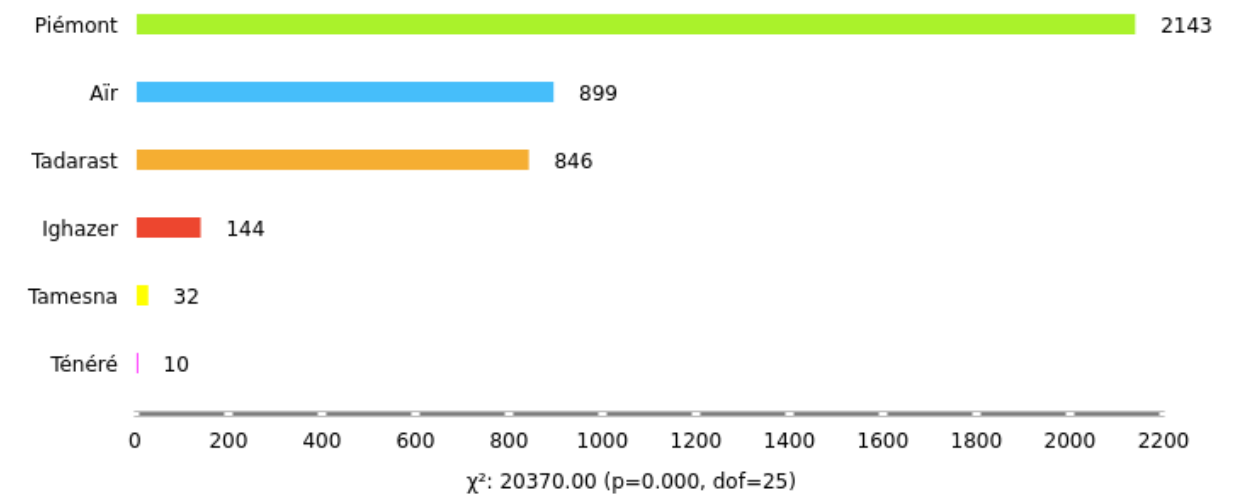
Figure 1: Nombre de monuments par zone géomorphologique
