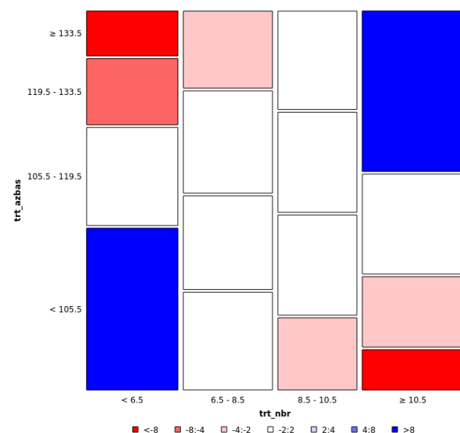
Figure 10: Mosaïque du nombre de tourette par rapport à l'azimut bas
