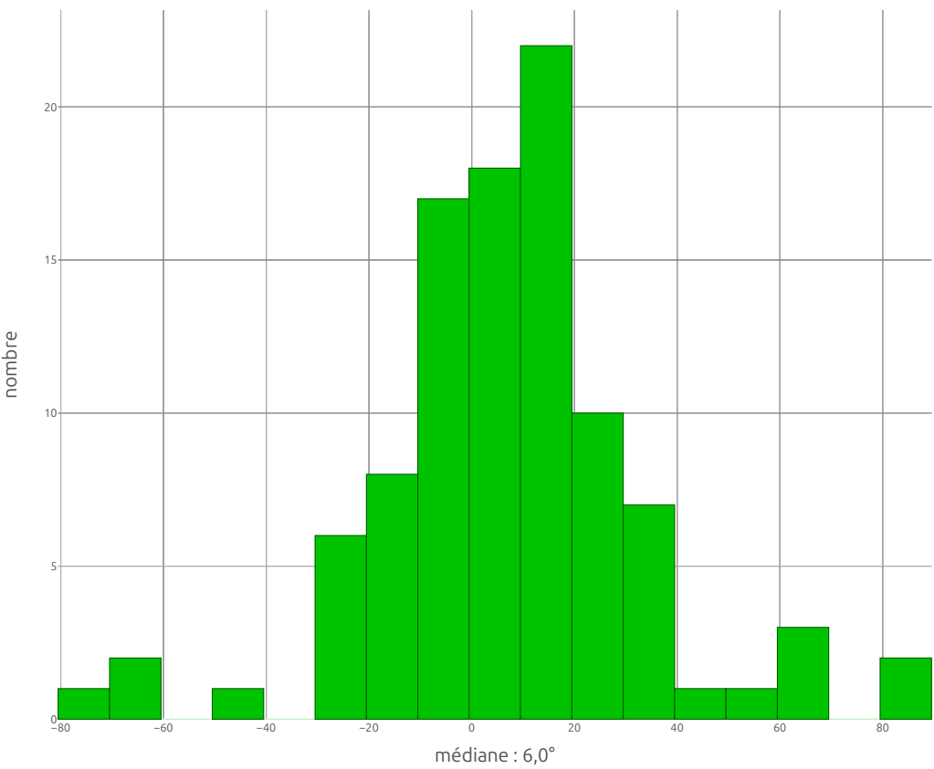
Distribution de l'azimut
